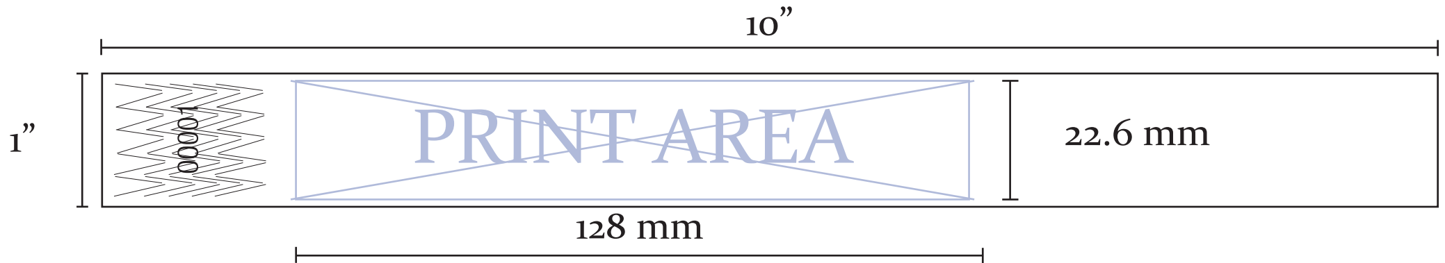
1" Tyvek Band
