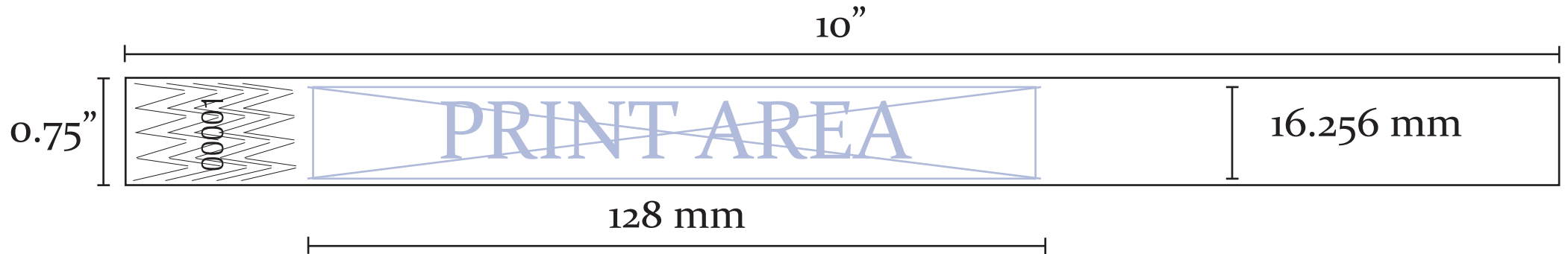
3/4" Tyvek Band
